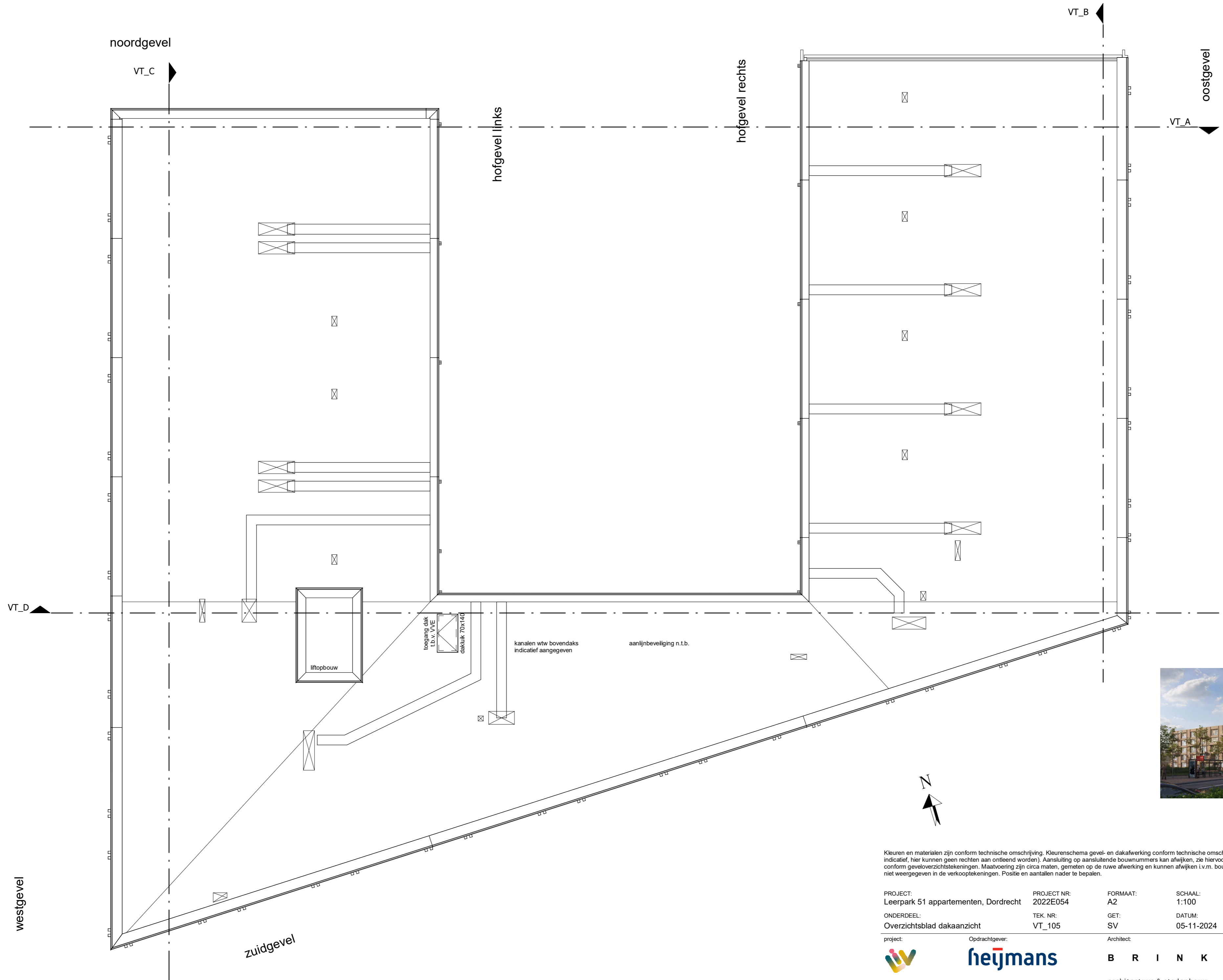
dakaanzicht
